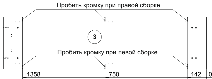
Схема 3. Подготовка отверстий
