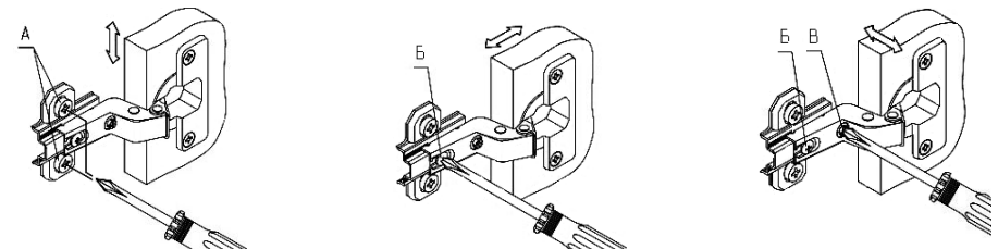
Схема 9. Регулировка положения фасада
