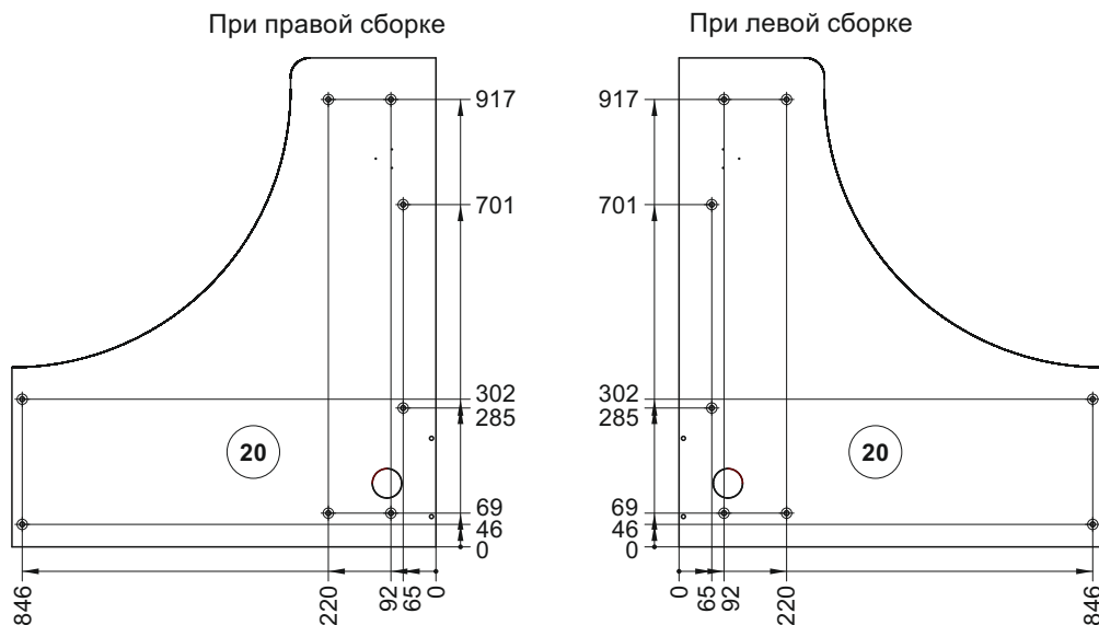
Схема 5. Сверление отверстий
