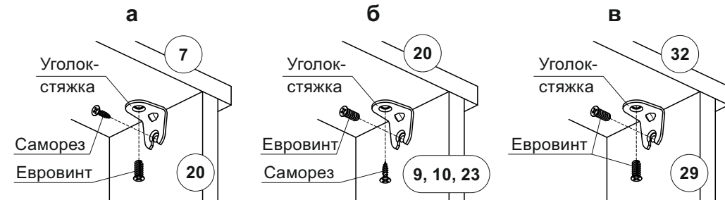
Схема 7. Установка уголка-стяжки
