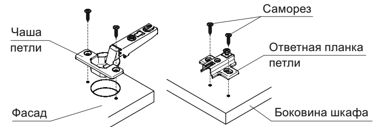
Схема 8. Установка петли
