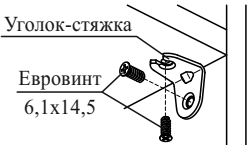
Схема 3. Установка уголка-стяжки
