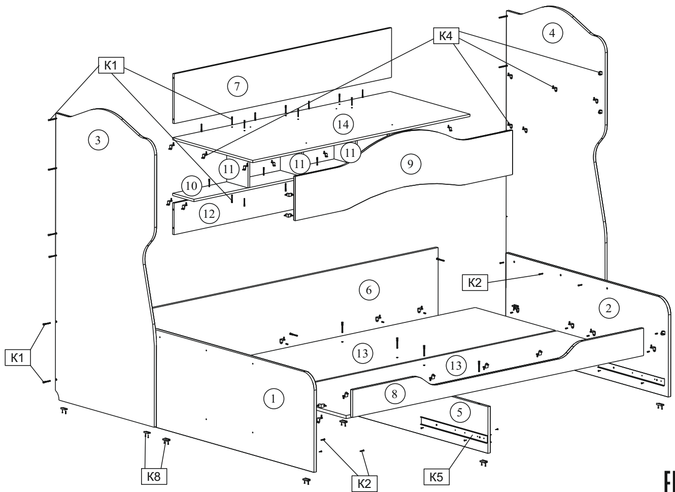
Схема 1. Сборка корпуса
