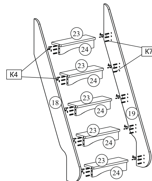
Схема 9. Сборка лестницы
