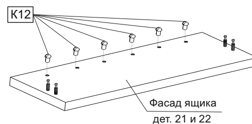
Схема 8.1. Установка держателя дна ящика
