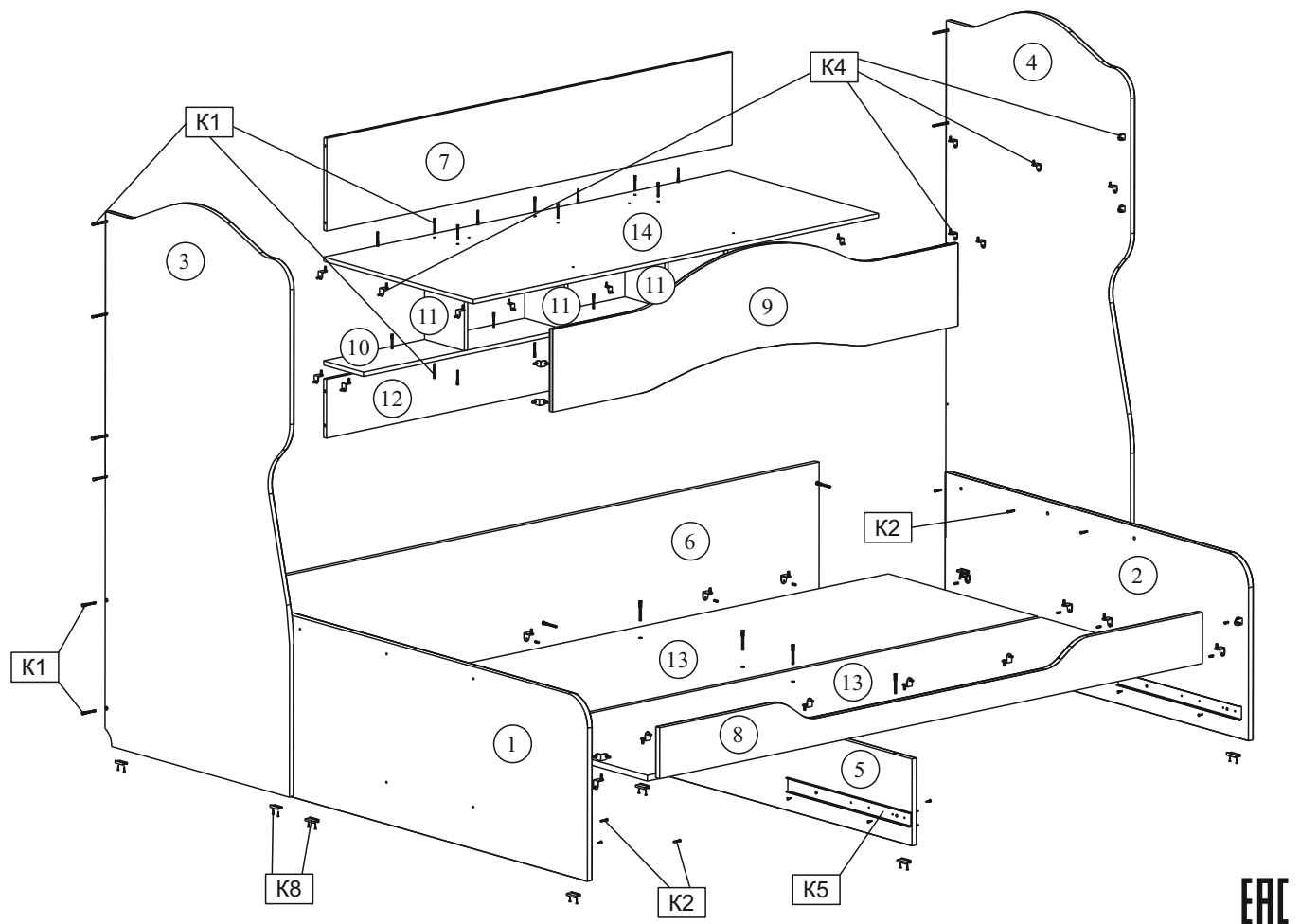
Схема 1. Сборка корпуса
