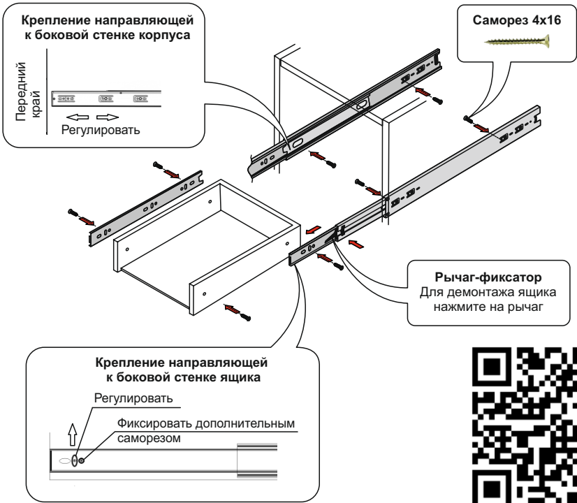
Схема 4. Установка ящика
