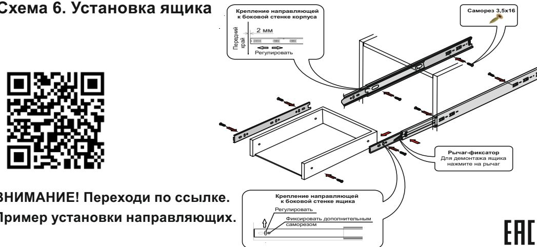
Схема 6. Установка ящика
