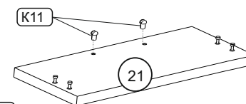
Схема 2.1. Установка держателей дна ящика
