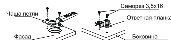
Схема 5. Регулирование зазоров и положения фасада.
